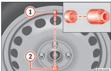
Fig. 54 Changement de roue : valve du pneu (1) et emplacement du boulon antivol de la roue (2).
