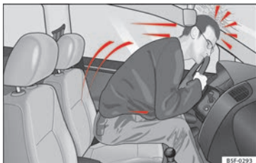
Fig. 70 Le conducteur n'ayant pas bouclé sa ceinture est projeté en avant.
