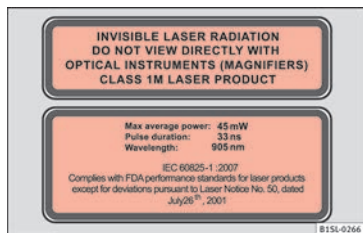
Fig. 163 Alertes relatives à l'utilisation du capteur laser de la fonction d'assistance au freinage en ville.
