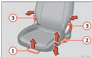
Fig. 13 Commandes du siège avant gauche.
