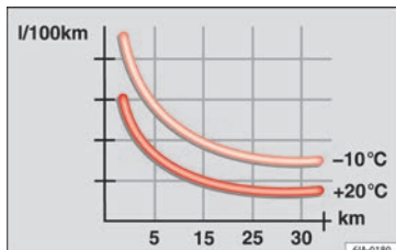
Fig. 150 Consommation de carburant en l/100 km à deux températures ambiantes différentes.
