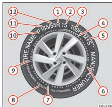
Fig. 178 Inscription universelle sur les pneus.
