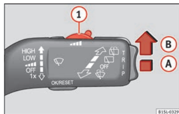
Fig. 114 Levier d'essuie-glace : réglage du détecteur de pluie ①.
