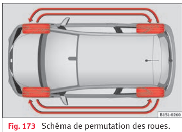
Fig. 173 Schéma de permutation des roues.
